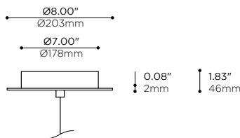
-R7 CANOPY OPTION (INTEGRATED DRIVER) OPTION DE PAVILLON -R7 (PILOTE INTÉGRÉ)
