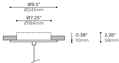
-FR7 RECESSED CANOPY OPTION (INTEGRATED DRIVER) OPTION DE PAVILLON ENCASTRÉ -FR7 (PILOTE INTÉGRÉ)
