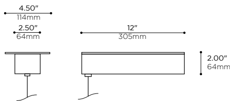
-S11 CANOPY OPTION (INTEGRATED DRIVER) OPTION DE PAVILLON -S11 (PILOTE INTÉGRÉ)
