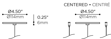
-R4 CANOPY OPTION (REMOTE DRIVER) OPTION DE PAVILLON -R4 (PILOTE À DISTANCE)
